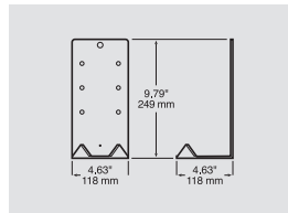
740-09 bracket
